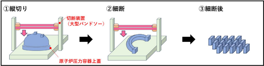
上蓋解体の流れ(概略)
