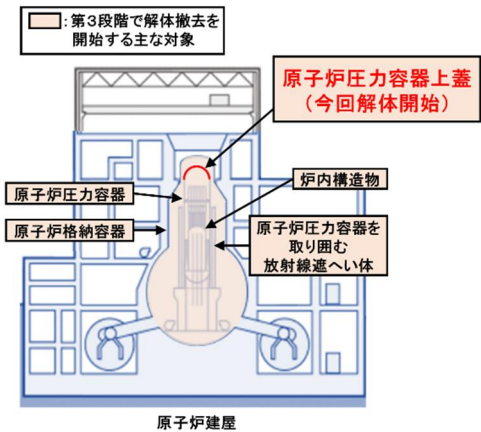
廃止措置第 3 段階の主な解体範囲
